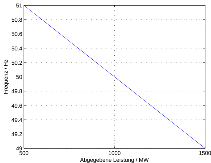
Abb. 4.1: f(P) -Kennlinie von Netz 1
