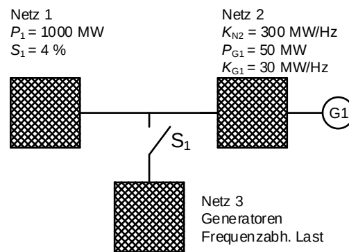
Abbildung 4. Verbundnetz aus drei Netzen
